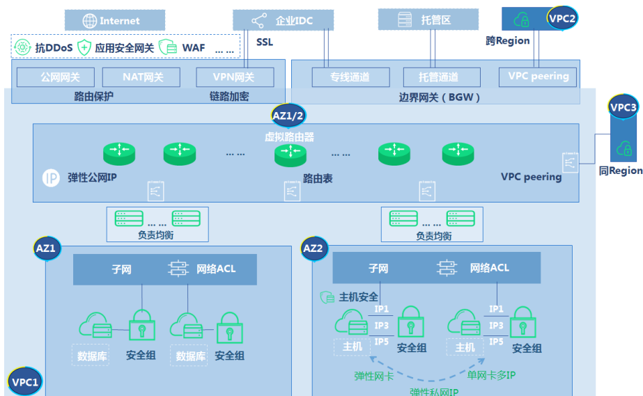
图 5 网络安全架构
