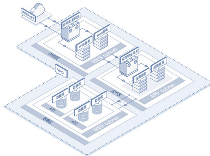
图 10 应用安全网关防护示意图
